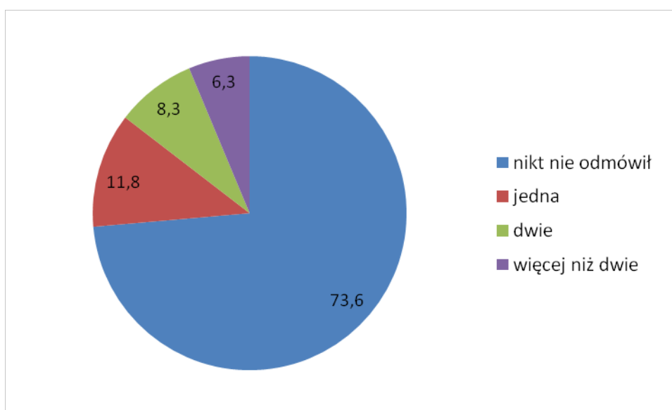
Rysunek 3.9. Liczba osób, które badany namawiał do wzięcia udziału w Badaniu RDS przed skutecznym przekazaniem zaproszeń (dane w %)
